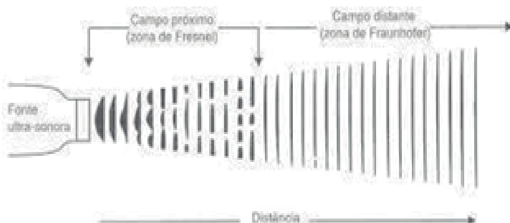
Figura 3: Feixe ultrassônico cilíndrico heterogêneo no campo próximo e tornando-se mais homogêneo no campo distante
