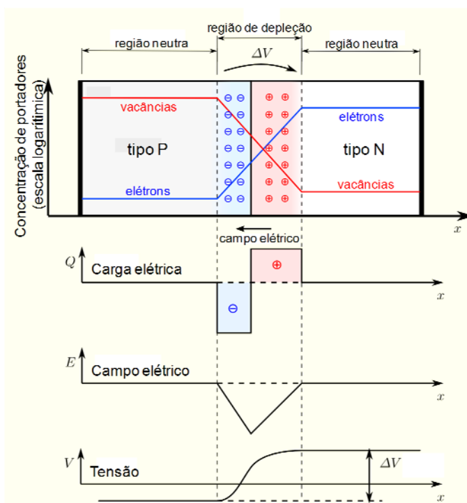
Figura 2 – Representação de um diodo (junção PN).
