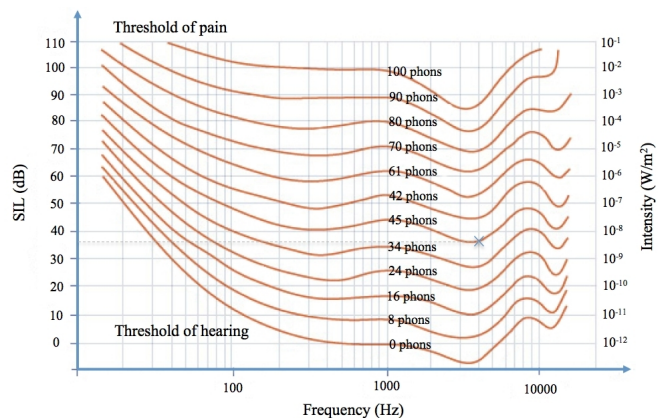
Figura 1: A escala decibel e a sensibilidade do ouvido humano.
