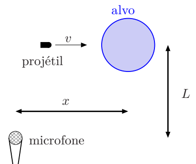
Figura 2: Dispositivo fotográfico de exposição rápida.
